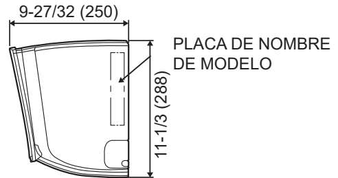
VISTA LATERAL
