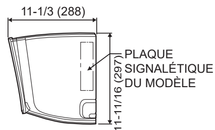
VUE LATÉRALE
