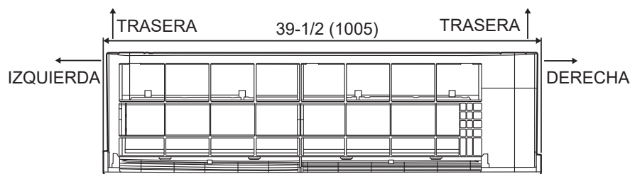
VISTA SUPERIOR
