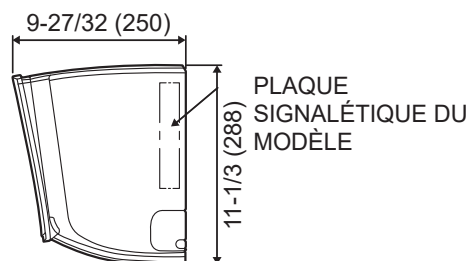
VUE LATÉRALE
